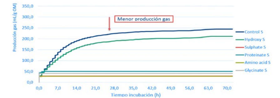
FIGURA 2. EVALUACIÓN IN VITRO: EFECTO DE LA FUENTE DE CU SOBRE LA PRODUCCIÓN DE GAS (ML/G MO)
